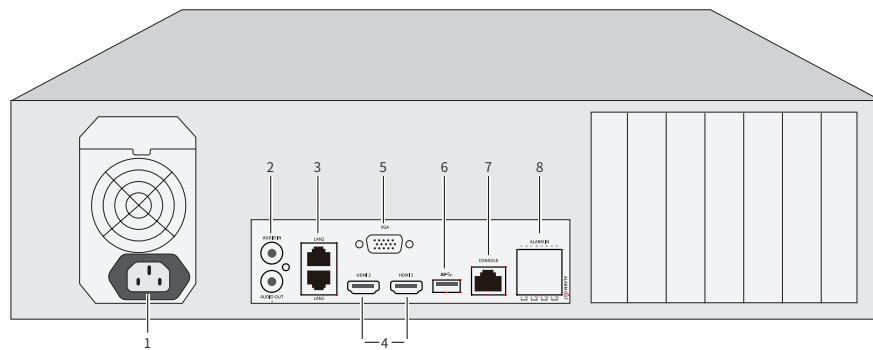
图1-3 TL-NVR7162-128后面板示意图
